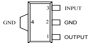
M4 Package (SOT-89)
